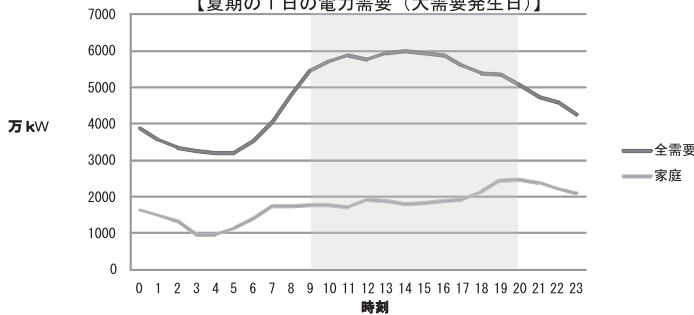
【夏期の1日の電力需要(大需要発生日)】
